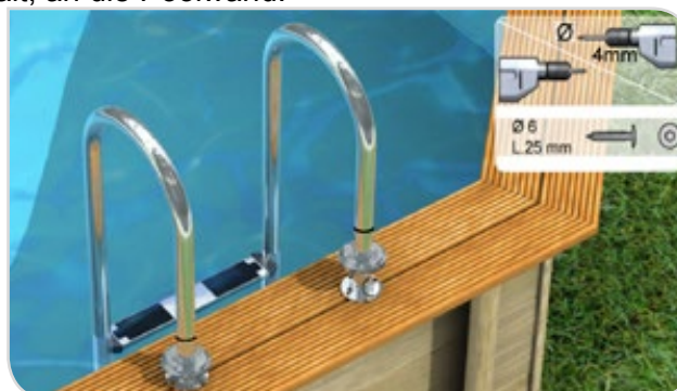
Abbildung 61 – Edelstahlleiter
